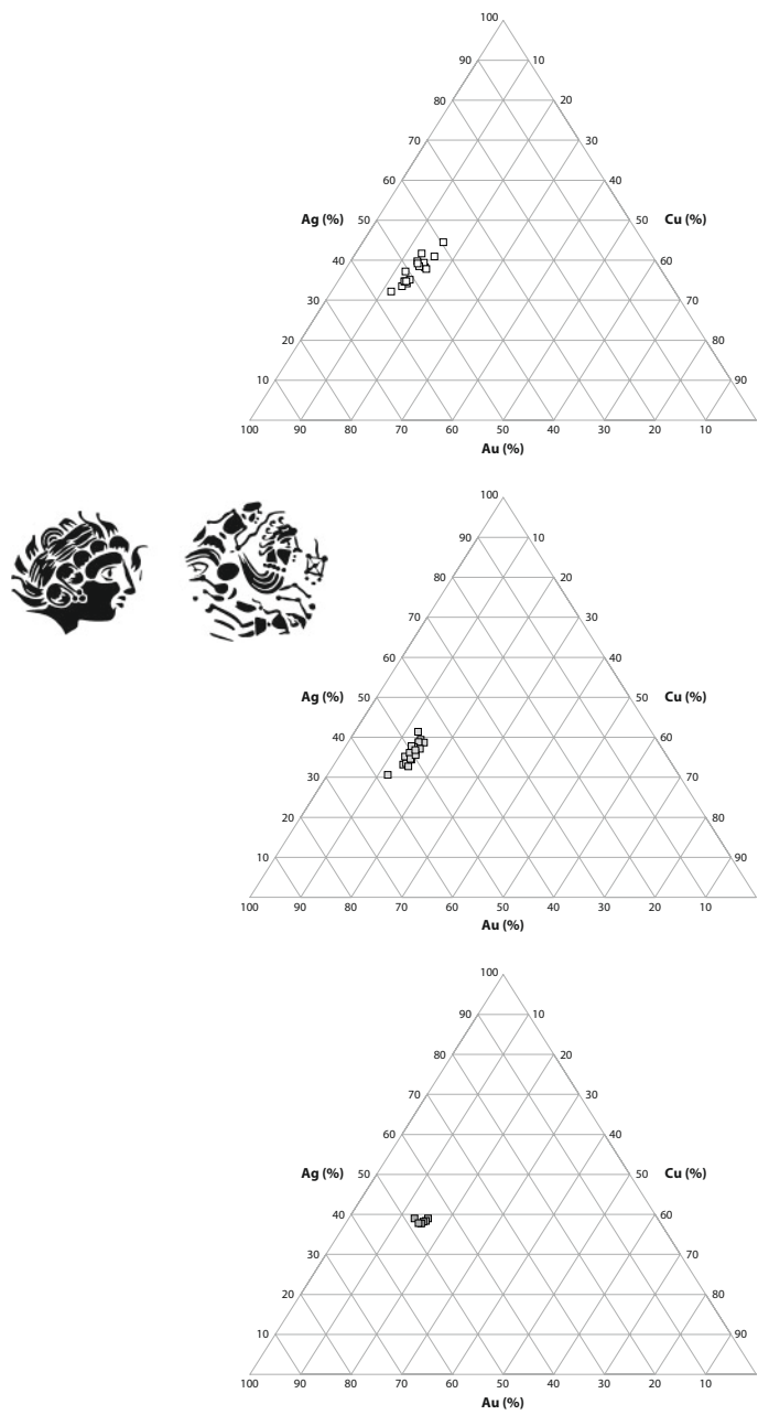
Figure 7 - Dépôt des Sablons, Le Mans : graphiques de composition métallique des chaînes 1, 2 et 4.
