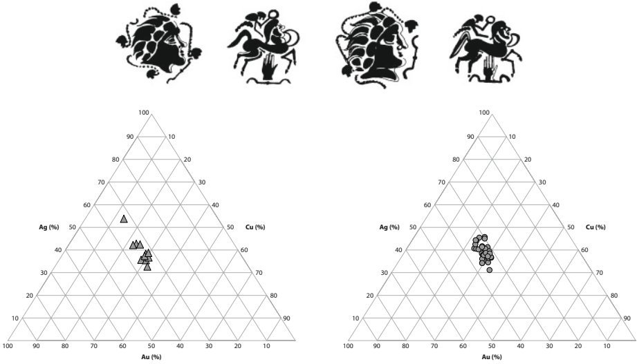
Figure 4 - Dépôt de Cheavanceaux : graphique de composition métallique de la série A : groupes KI et KII.
