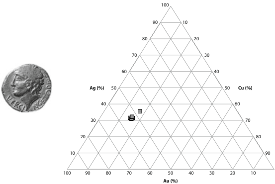
Figure 6 - Statères de Vercingétorix : graphique de composition métallique (série1B1).
