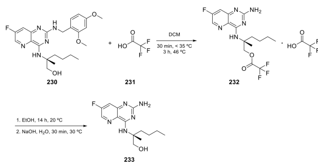
Scheme 23. (2S)-2-((2-amino-7-fluoropyrido[3,2-d]pyrimidin-4-yl)amino)-2-methylhexan-1-ol ( 233 ) [73].
