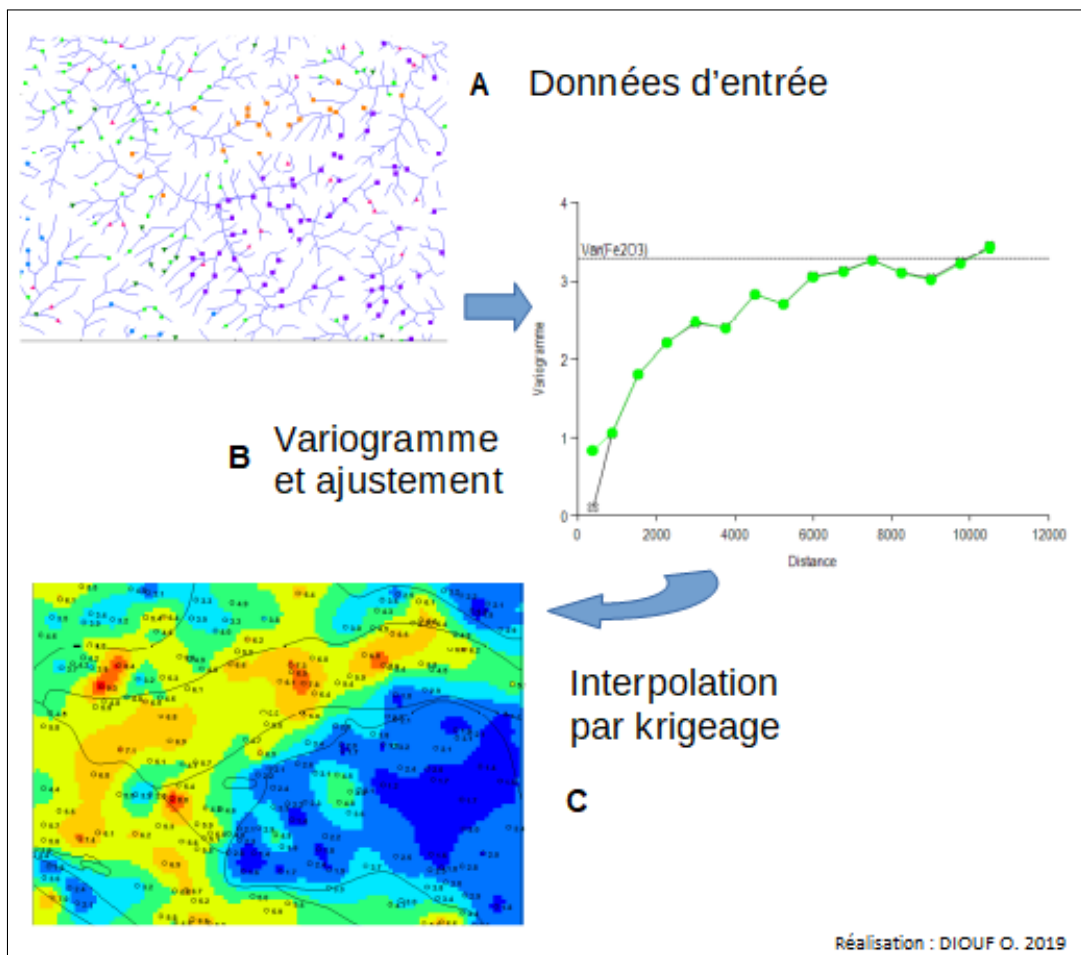
SCHÉMA 1.1 – Processus de traitement géostatistique A. Données ponctuelles localisées, B. Variogramme et ajustement des paramètres (modèle), C. Cartographie krigée
